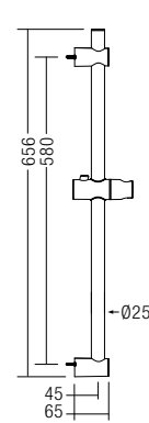
AMBA-803 SUS 304 Shower Rail Only (ABS Holder) Round • Stainless Steel SUS 304 • Black • 1 pc/box, 12 pcs/ctn RM223.00
